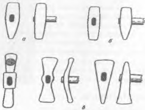
Мал. 4. Форми молотків:
