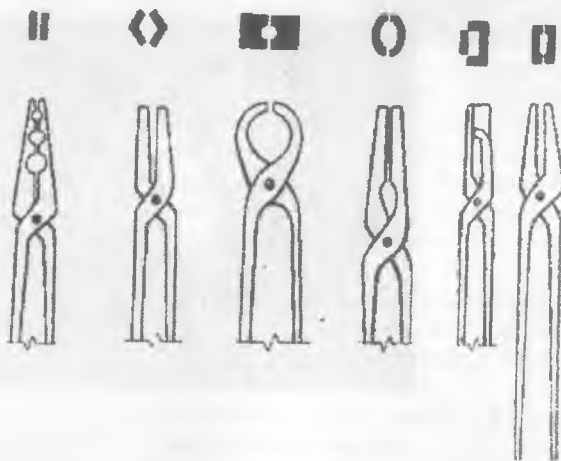
Мал. 5. Форми губок ковальських кліщів для утримування заготовок різної форми та перерізів.
